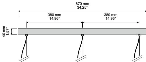
3A Dreifachaufhängung 3A triple suspension
