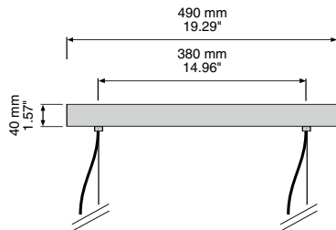
2A Doppelaufhängung 2A double suspension
